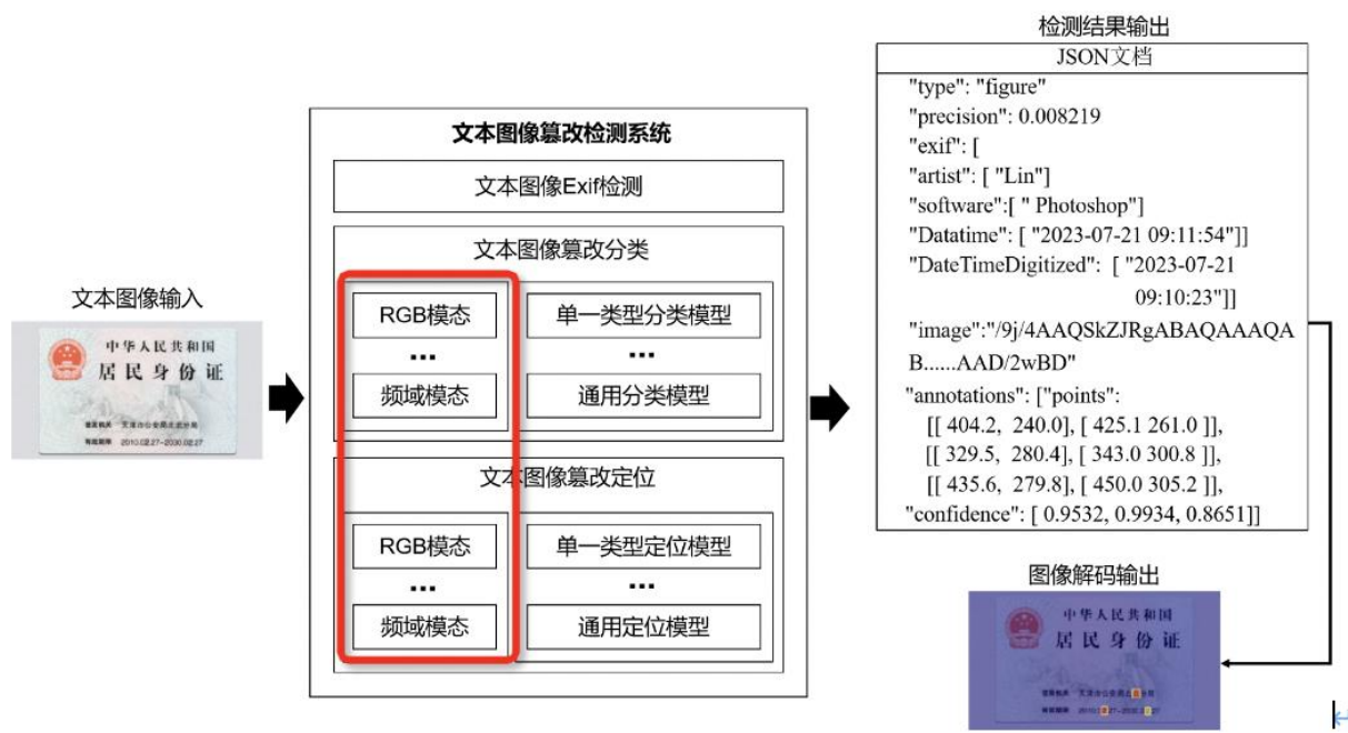
图12、文本图像篡改检测系统流程
