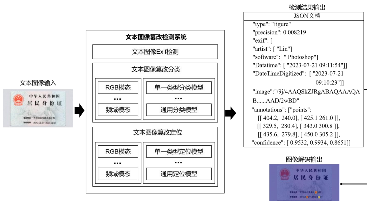
图 13 文本图像篡改检测系统流程
