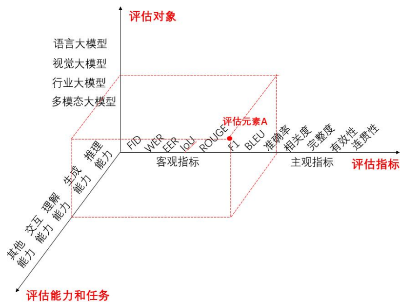
图 2 评估框架
